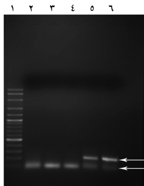
شکل ۵ محصول RT-PCR الکتروفورز شده در ژل آگارز؛ چاهک ۱ نشانگر، چاهک ۲ نمونه کنترل منفی، چاهک ۳ ژن بتا اکتین تحت تأثیر ۵۰۰ میلی گرم بر میلی لیتر عصاره شیرین بیان، چاهک ۴ ژن بتا اکتین (کنترل)، چاهک ۵ ژن afIR تحت تأثیر ۵۰۰ میلی گرم بر میلی لیتر عصاره شیرین بیان، چاهک ۶ ژن afIR (کنترل)
