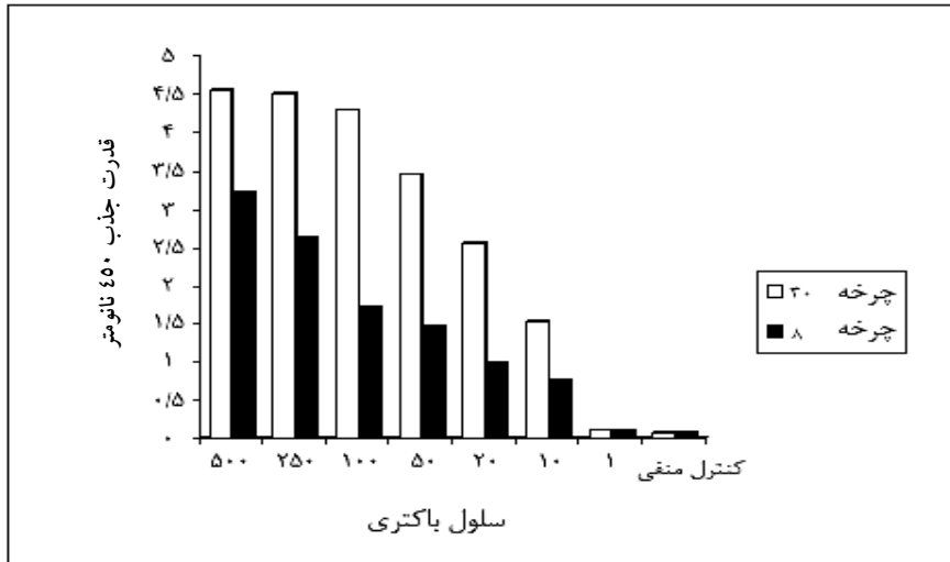
نمودار ۱ تعیین حساسیت روش PCR-ELISA با استفاده از نمونه سلول باکتری سالمونلا تیفی موربیوم
