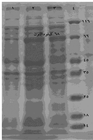
شکل ۴ ارزیابی بیان UreB 332 -HpaA نوترکیب در میزبان بیانی E. coli , BL-21(DE3) روی SDS-PAGE (ستون ۱) لیزات باکتریایی حاصل از یک کلون نوترکیب القا نشده (کنترل بیان)، ستون‌های ۲ و ۳) لیزات باکتریایی حاصل از ۲ کلون نوترکیب القا شده با IPTG و بیان UreB 332 -HpaA نوترکیب (۶۸ کیلودالتون)
