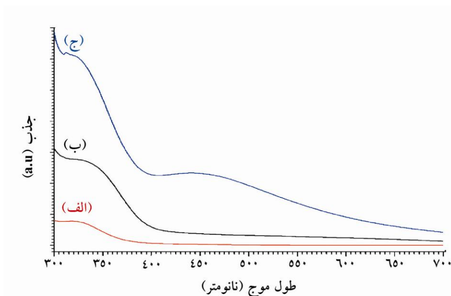
شکل ۳ جذب اسپکتروفتومتری UV-Vis؛ (الف) نیترات نقره، (ب) عصاره قارچ دنبلان، (ج) نانوذرات نقره
