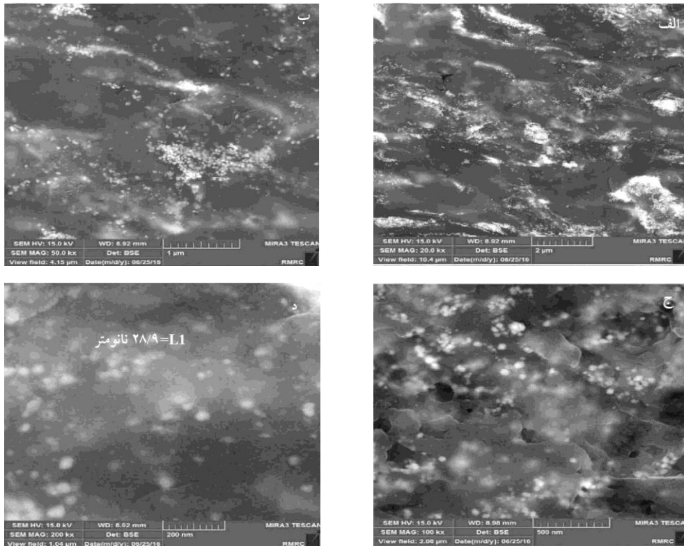
شکل ۶ تصاویر FESEM نانوذرات سنتز شده از عصاره آبی قارچ دنبان
