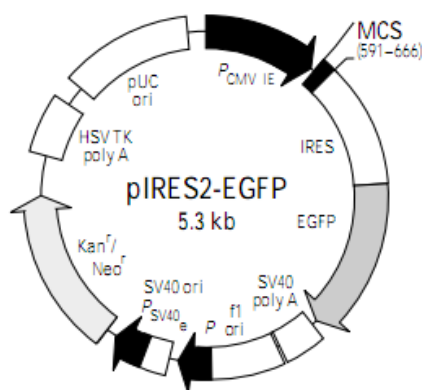
شکل ۱ ناقل pIRES2-EGFP
