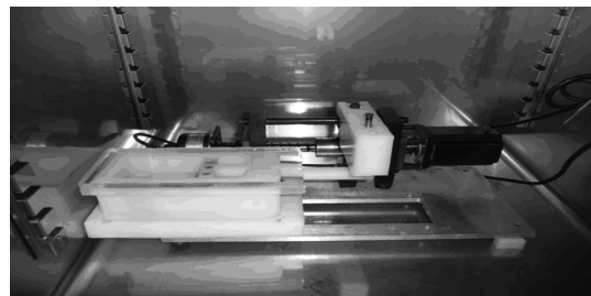
شکل ۲ محفظه کشت سلول و بخش الکترومکانیکی کنترل حرکت آن داخل انکوباتور
