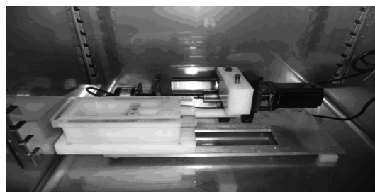
شکل ۲ محفظه کشت سلول و بخش الکترومکانیکی کنترل حرکت آن داخل انکوباتور
