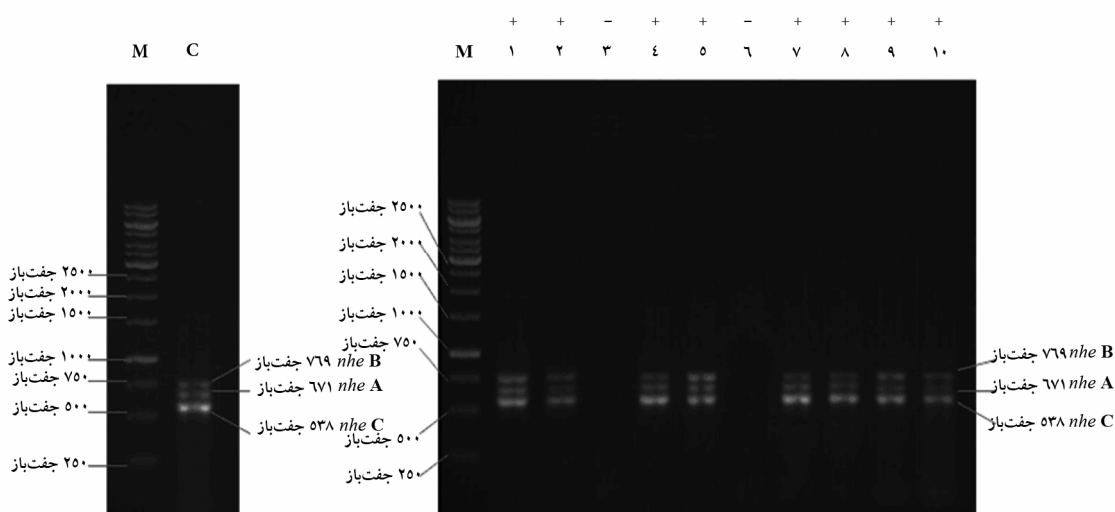
شکل ۲ نتیجه الکتروفورز مربوط به PCR چندگانه با آغازگرهای ژن‌های nheC nheB nheA برای باسیلوس سرئوس‌های جدا شده از ده نمونه برنج پخته شده است. برای نمونه‌های شماره ۳ و ۶ باندها مشاهده نشد. (M) نشانگر ۱ کیلوبازی، (C) کنترل مثبت
