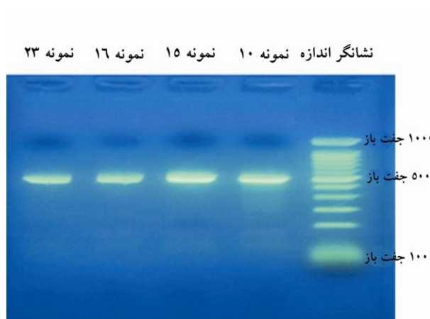
شکل ۱ الکتروفورز محصولات PCR ژن ERG11 کاندیدا آلیکس مقاوم به فلوکونازول، روی ژل آگارز ۱/۵ درصد رنگ آمیزی شده با Gel-red؛ از راست به چپ (۱) نشانگر اندازه (M100)، (۲) DNA شماره ۱۰، (۳) DNA شماره ۱۵، (۴) DNA شماره ۱۶، (۵) DNA شماره ۲۳
