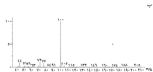
شکل ۳ کروماتوگرام کپسول لاغری Fat loss (الف) و طیف جرم آمفیرامون (ب) با استفاده از GC-MS
