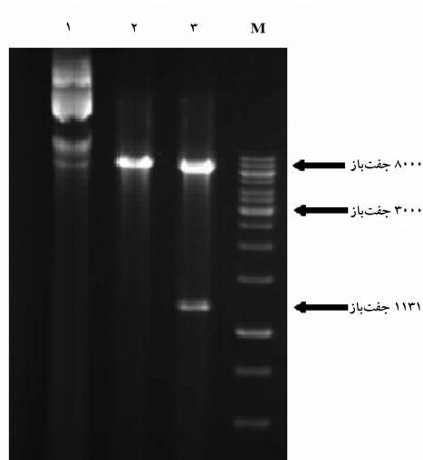
شکل ۲ تأیید درستی پلاسمید pGL3/Oct4 promoter/TK با روش هضم تک آنزیمی و دو آنزیمی؛ (M) DNA نشانگر، (۱) پلاسمید pGL3/Oct4 promoter/TK هضم شده با آنزیم های EcoRI و BamHI ، (۲) پلاسمید pGL3/Oct4 promoter/TK هضم شده با آنزیم BamHI ، (۳) پلاسمید pGL3/Oct4 promoter/TK
