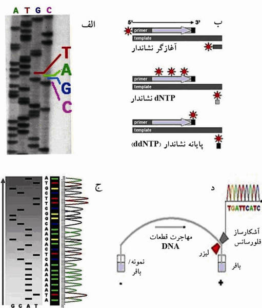
شکل ۲ الف) قسمتی از رادیوگرافی ژل قطعات تعیین توالی شده نشاندار (ب) آغازگرها با فلورسنت یا رادیو اکتیو نشانه‌گذاری می‌شوند و در نهایت قطعه DNA با dNTP یا ddNTP نشاندار می‌شود (ج) نقاط اوج (Peaks) فلورسنت در مقایسه با باندهای رادیو اکتیو (د) الکتروفورز موینه‌ای
