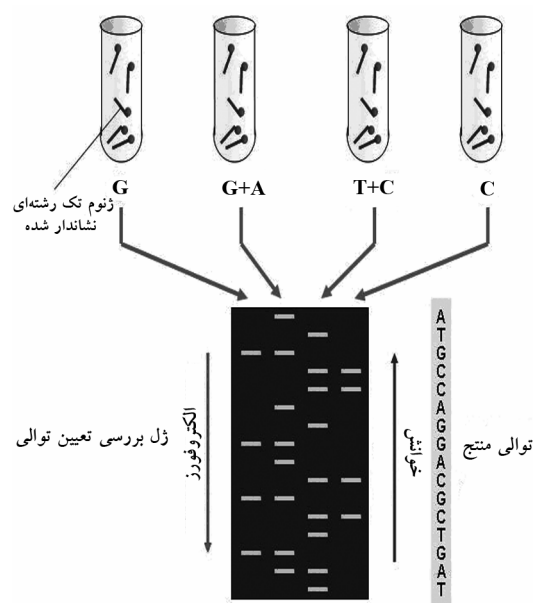
شکل ۱ روش تعیین توالی ماکسام-گیلبرت
