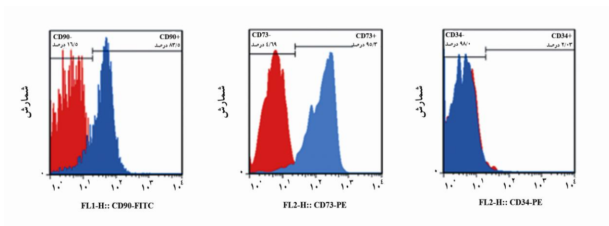
شکل ۲ آنالیز فلوسایتومتری به‌منظور تأیید هویت سلول‌های بنیادی مزانشیمی؛ آنالیز فلوسایتومتری بیان مثبت نشانگرهای سطحی CD90 و CD73 و فقدان بیان آنتی‌ژن CD34 را برای سلول‌های بنیادی مزانشیمی نشان داد که نشانگر درستی جداسازی سلول‌های بنیادی مزانشیمی از مغز استخوان است.
