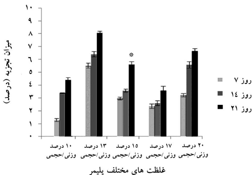
شکل ۳ نتایج حاصل از میزان تخریب داربست‌های PLA الکتروریسی شده در غلظت‌های مختلف؛ غلظت PLA ۱۵ درصد حجمی/وزنی (*) تفاوت معنی‌داری با دیگر غلظت‌های این گروه دارد ( P < 0.05 ) (میانگین داده‌ها \pm SE ).
