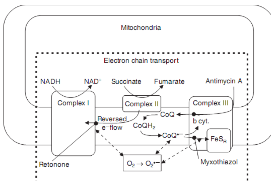
شکل ۱ نقاط ممکن تولید ROS درون زنجیره انتقال الکترون [۲۸]: \text{CoQH} = \text{کوآنزیم Q} , \text{CoQH}_2 = \text{کوآنزیم احیا شده Q} , \text{CoQ}^- = \text{کوآنزیم اکسید شده Q} , \text{FeS}_R = \text{پروتئین سولفور-آهن ریسکه (Rieske iron)}
