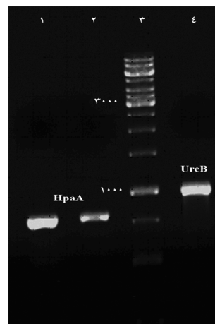
شکل ۱ الکتروفورز محصول PCR ژن‌های hpaA و ureB از ژنوم هلیکوباکتر پیلوری روی ژل آگارز ۱ درصد؛ ستون ۱ (۲) محصول PCR برای ژن hpaA با اندازه ۸۵۰ جفت‌باز، ستون ۳ (۴) نشانگر وزن مولکولی ۱۰۰۰ جفت‌بازی، ستون ۴) محصول PCR برای قطعه ژنی ureB332 با اندازه ۱۰۱۷ جفت‌باز
