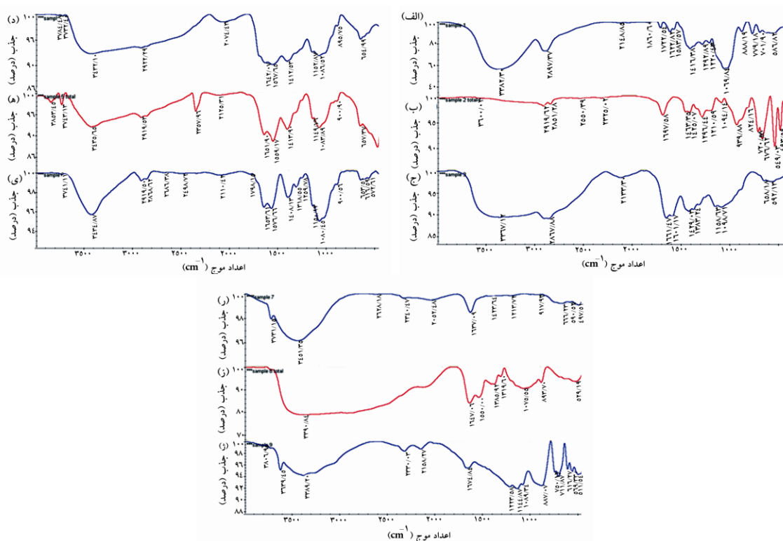
شکل ۳ اسپکترومتری FT-IR از (الف) DOX، (ب) میریستات، (ج) CS، (د) MCS، (ه) MCS-DOX بدون سونیکاسیون، (ی) MCS-DOX با سونیکاسیون، (ر) PCS-DOX (ز)، PCS، TPP
