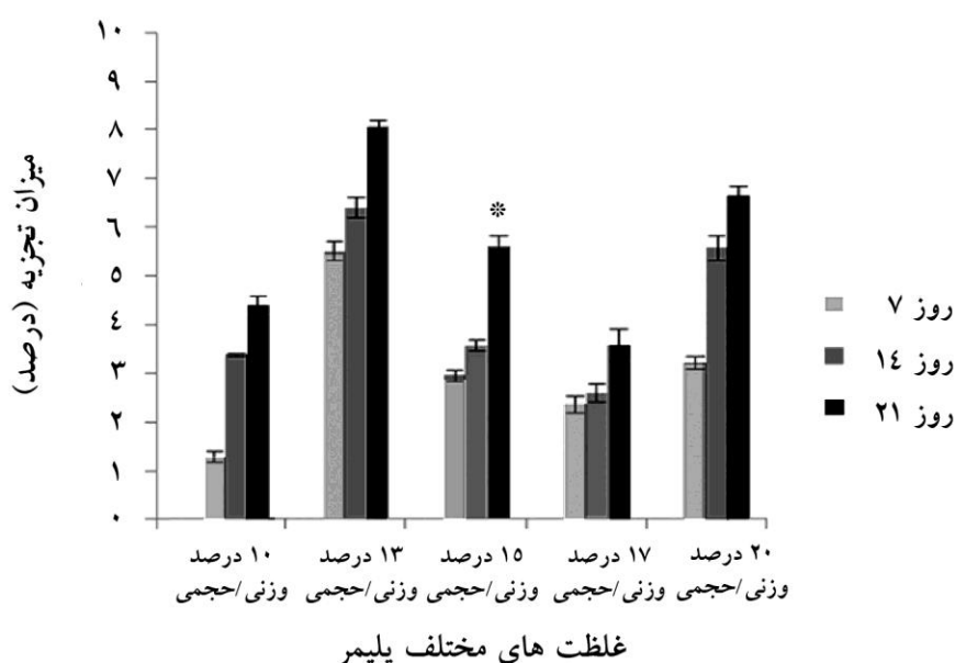
شکل ۳ نتایج حاصل از میزان درصد تخریب داربست‌های PLA الکتروریسی شده در غلظت‌های مختلف؛ غلظت PLA ۱۵ درصد حجمی/وزنی (*) تفاوت معنی‌داری با دیگر غلظت‌های این گروه دارد ( P < 0.05 ) (میانگین داده‌ها \pm SE ).
