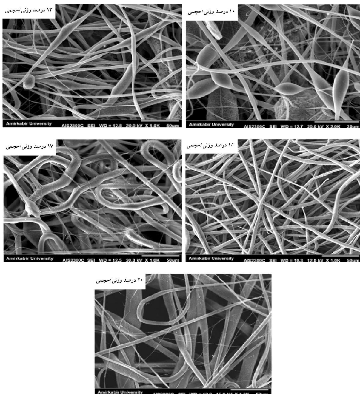
شکل ۱ تصاویر SEM از داربست‌های الکتروریسی شده PLA به روش الکتروریسی مرطوب در غلظت‌های مختلف
