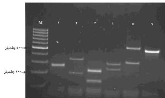
شکل ۲ الگوی الکتروفورزی PCR-RFLP با آنزیم MspI روی ژل آگارز؛ (M) نشانگر مولکولی ۱۰۰ جفت‌بازی، چاهک ۱) کانیدیدا کروزئی، چاهک ۲) کانیدیدا تروپیکالیس، چاهک ۳) کانیدیدا (مچنیکوویا) پولچریم، چاهک ۴) کانیدیدا آلیکنس، چاهک ۵) کانیدیدا گلابراتا و چاهک ۶) کانیدیدا پاراپسیلوزیس
