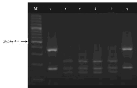
شکل ۳ الکتروفورز محصولات PCR بعد از هضم اندونوکلازی (RFLP) با آنزیم MboI برای افتراق گونه دابلینسیس از آلیکنس؛ (M) نشانگر مولکولی ۱۰۰ جفت‌بازی، چاهک ۱) کانیدیدا دابلینسیس (سویه استاندارد شماره ۷۹۸۷)، چاهک‌های ۲-۵) کانیدیدا آلیکنس (سویه‌های جدا شده از بیماران) و چاهک ۶) کانیدیدا دابلینسیس (سویه استاندارد شماره ۷۹۸۸)
